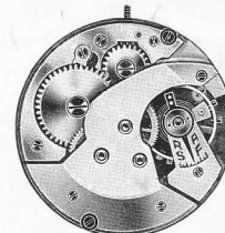
11 1/2''' cal. 1294
